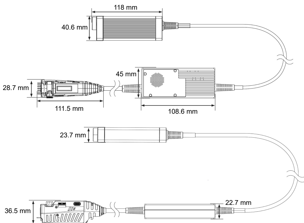
图 4.2 探头尺寸
