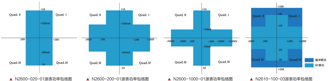
▲ N2600-020-01源表功率包络图
