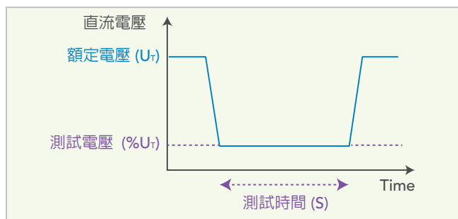
直流輸入電壓抗擾度測試
