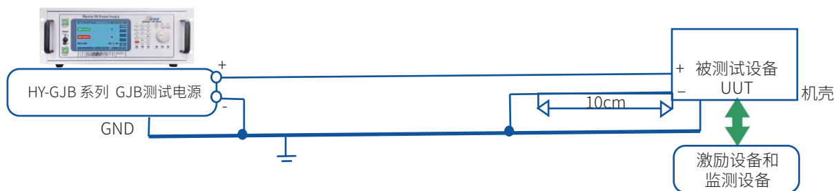
图LDC302-1 非正常电压瞬变试验系统典型配置
