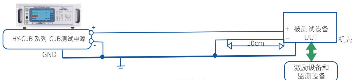
图LDC104-1 脉动试验系统典型配置
