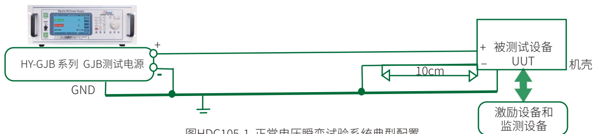
图HDC105-1 正常电压瞬变试验系统典型配置
