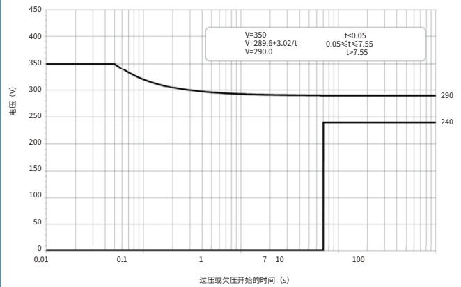
GJB 181B-2012 图17 270V直流非正常工作电压极限
