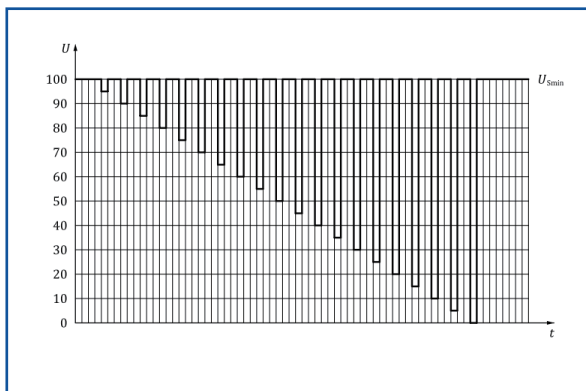
图12-电压降下复位行为的测试曲线
