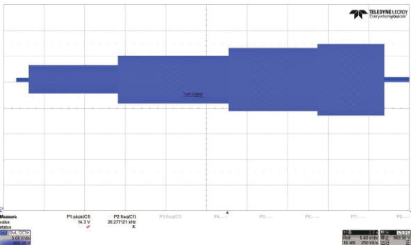
DC900V包络线
