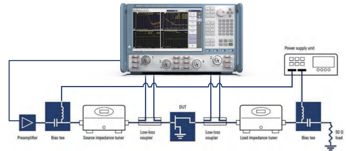
负载牵引测试示意图
