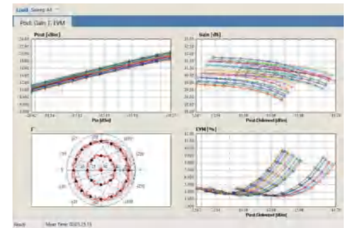
扫描互调失真扫描类型
