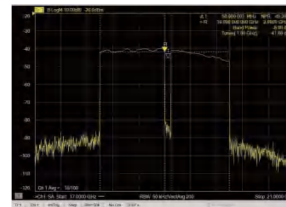
信号校准前
